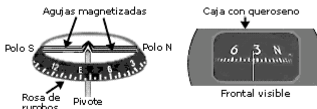
Fig.2.9.4 - Componentes de una brújula.
