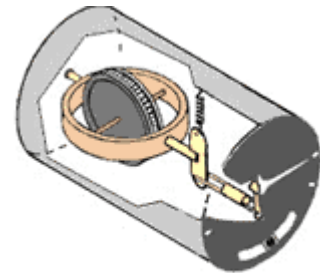
Fig.2.8.3 - Coordinador de viraje.
