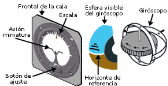
Fig.2.6.2 - Componentes del horizonte artificial.
