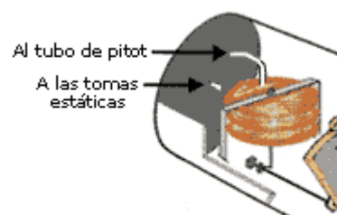
Fig.2.5.2 - Construcción anemómetro.
