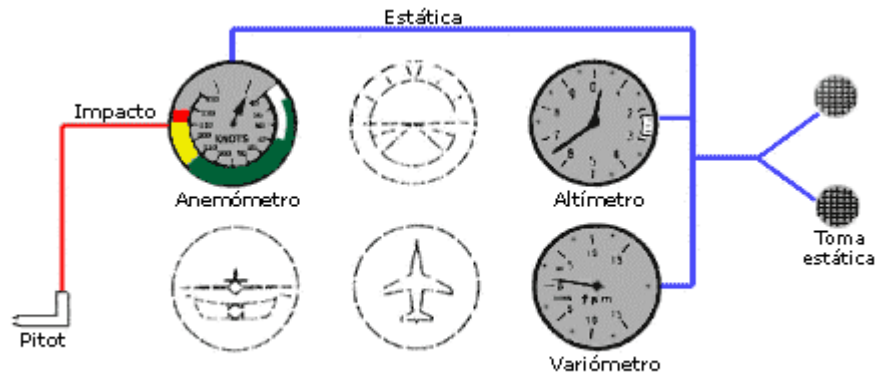
Fig.2.2.2 - Sistema de pitot y estática.
