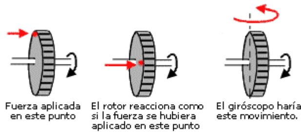
Fig.2.2.4 - Precesión giroscópica.
